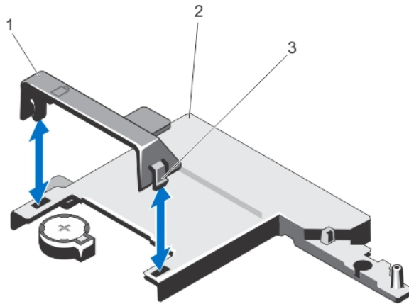
그림 34. 시스템 배터리 분리
