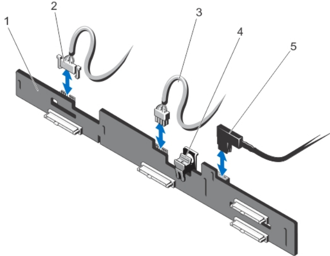
그림 36. 2.5 인치 (x4) 하드 드라이브 후면판 분리 및 설치
