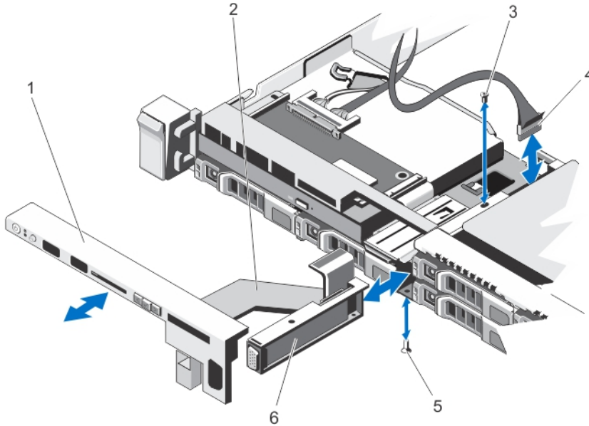
그림 40. VGA 모듈 분리 및 설치
