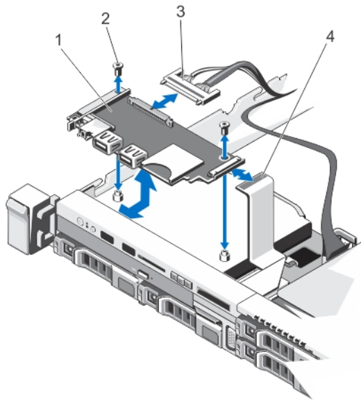
그림 38. 제어판 보드 분리 및 설치
