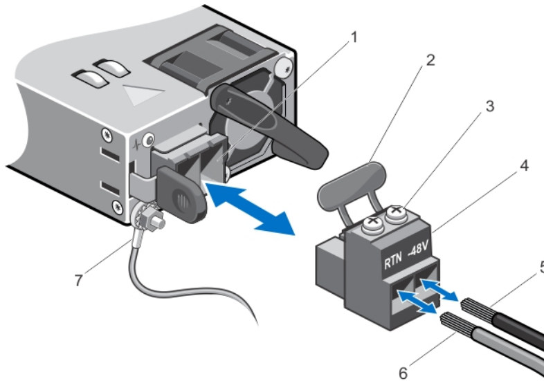
그림 31. DC 입력 전선 조립
