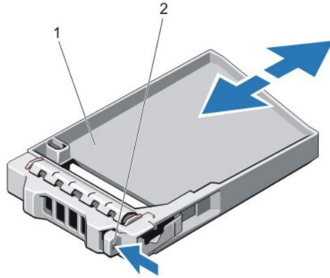
그림 14. 2.5 인치 하드 드라이브 보호물 분리 및 설치
