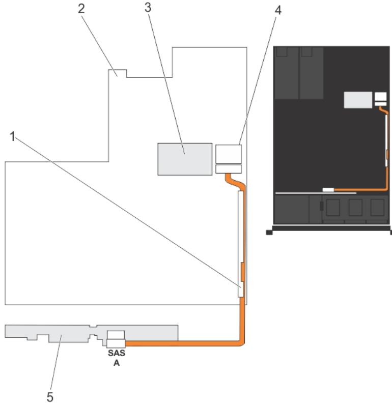
그림 37. 케이블 연결 다이어그램 - 2.5 인치 (x4) 시스템
