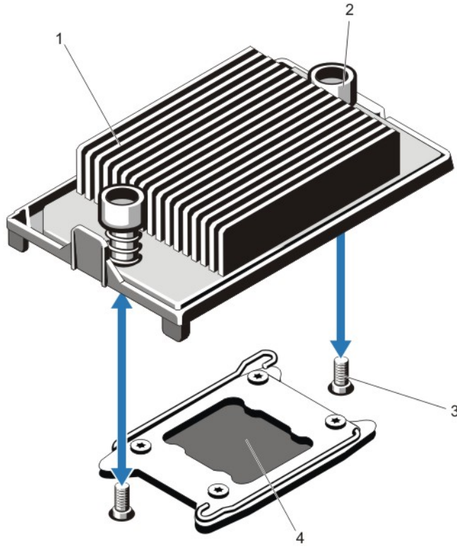
그림 26. 방열판 분리 및 설치
