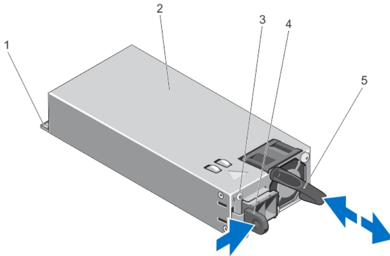
그림 32. DC 전원 공급 장치 분리 및 설치
