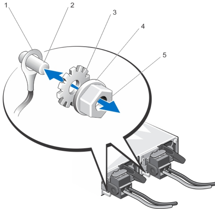
그림 30. 안전 접지선 조립 및 연결
