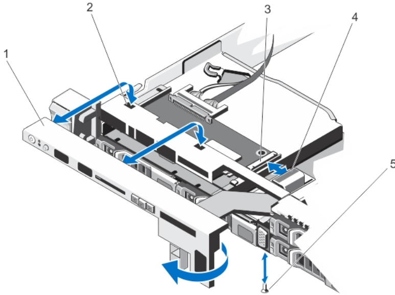
그림 39. 제어판 분리 및 설치
