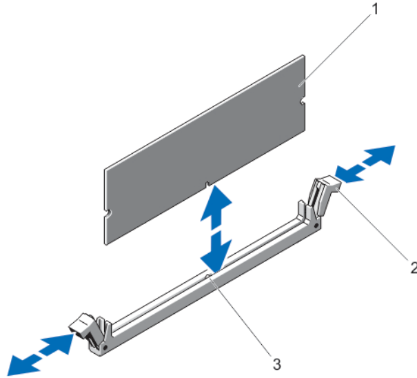
그림 13. 메모리 모듈 분리 및 설치
