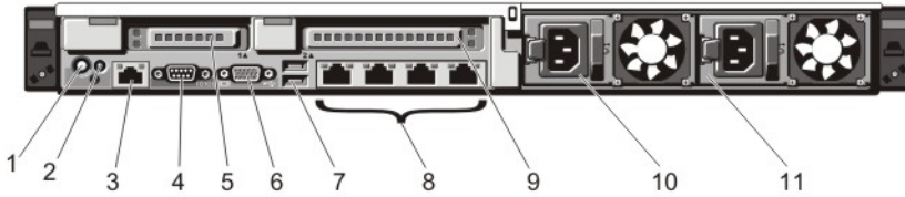
그림 4. 후면 패널 구조 및 표시등
