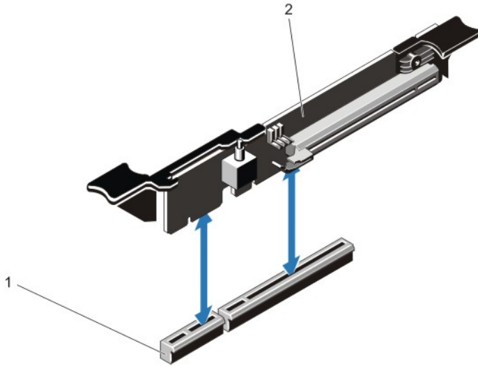
그림 22. 확장 카드 라이저 3 분리 및 설치
