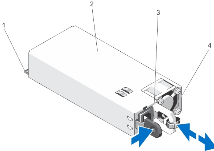
그림 29. AC 전원 공급 장치 분리 및 설치
