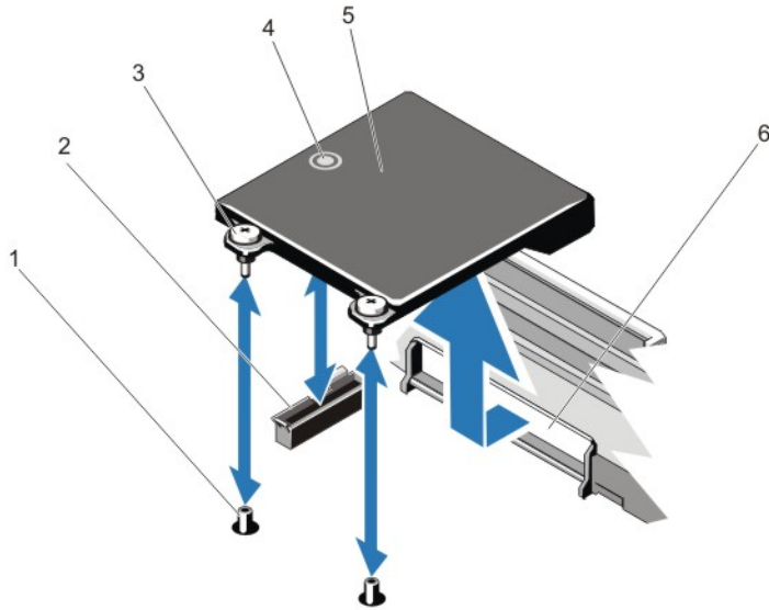
그림 25. 네트워크 도터 카드 분리 및 설치
