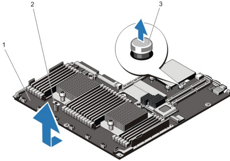
그림 41. 시스템 보드 분리 및 설치
