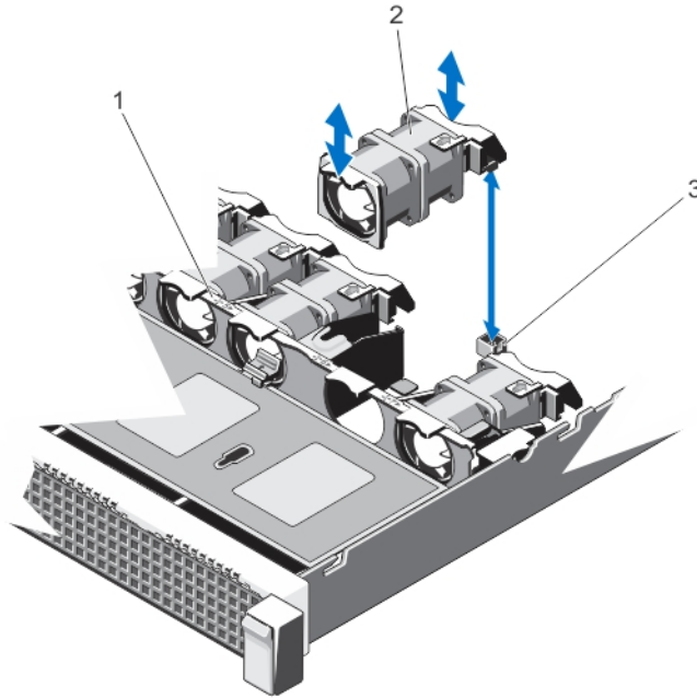
그림 18. 냉각 팬 분리 및 설치
