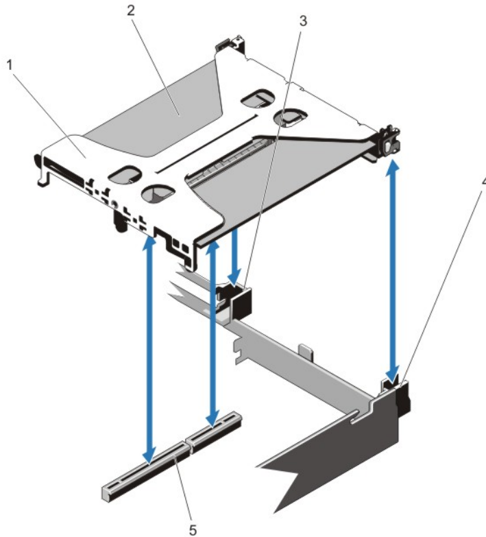
그림 21. 확장 카드 라이저 1 분리 및 설치
