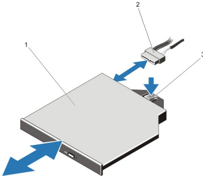
그림 17. 광학 드라이브 분리 및 설치
