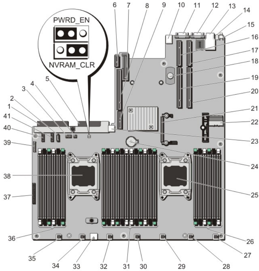
그림 42. 시스템 보드 커넥터 및 점퍼
