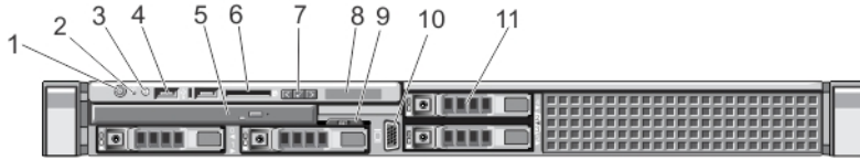
그림 1. 전면 패널 구조 및 표시등
