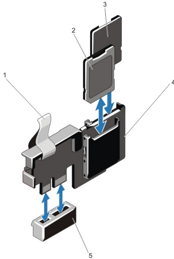
그림 24. 내부 이중 SD 모듈 분리 및 설치
