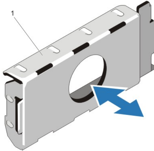
그림 33. 전원 공급 장치 보호물 분리 및 설치
