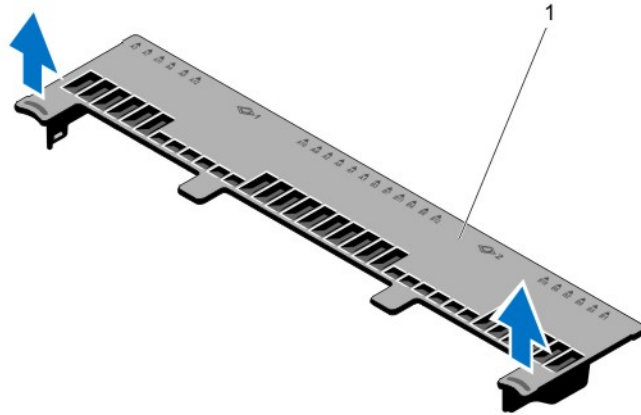
그림 11. 냉각 덮개 분리 및 설치
