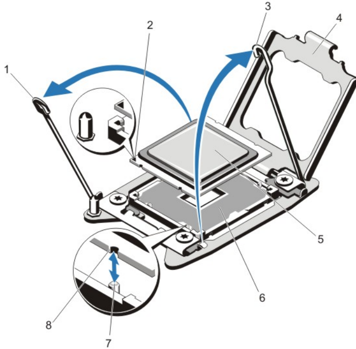
그림 28. 프로세서 분리 및 설치
