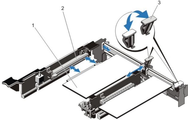
그림 20. 확장 카드 분리 및 설치
